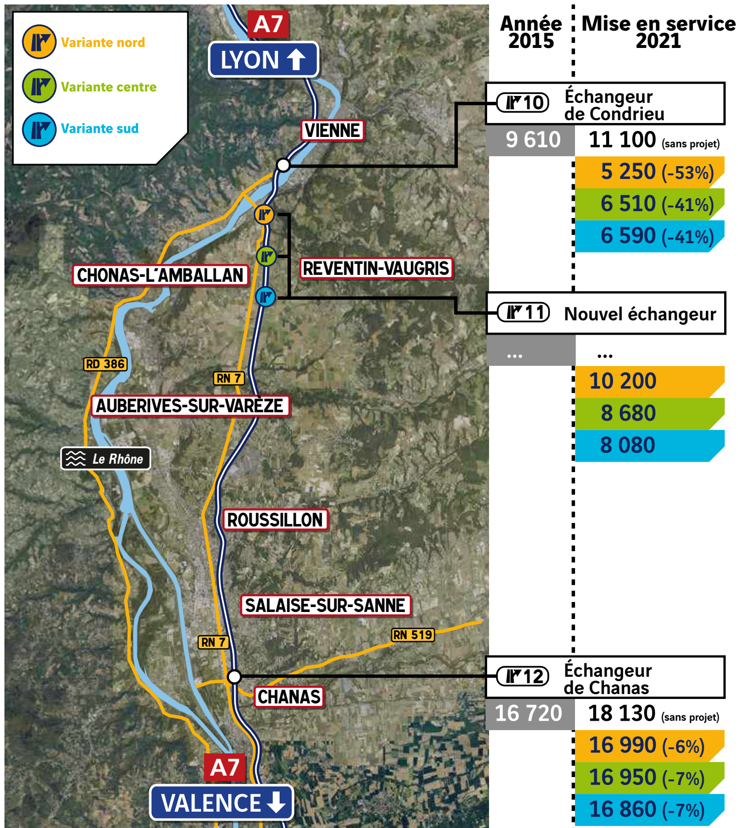
Trafic moyen journalier annuel (TMJA) exprimé en nombre de véhicules par jour.
