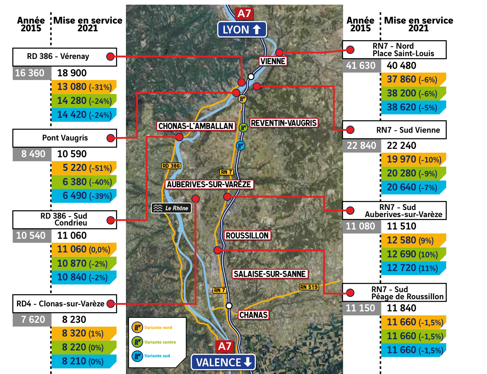
Trafic moyen journalier annuel (TMJA) exprimé en nombre de véhicules par jour.
